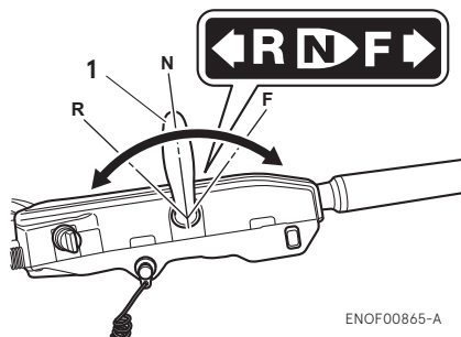
1. Levier inverseur
